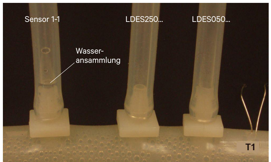
Bild 5 Verbindungsschläuche ~10 s nach Beginn von Test #1
