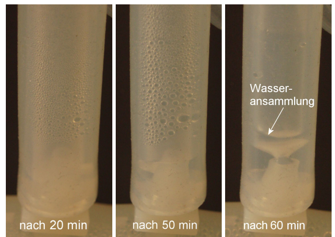
Bild 7 Verstopfung des 1/4 inch-Verbindungsschlauchs zum Sensor 1-1 während Test #2
