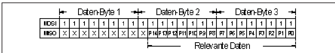
Bild 5: 3-Byte-Datenübertragung eines 15 Bit langen Druckwertes
