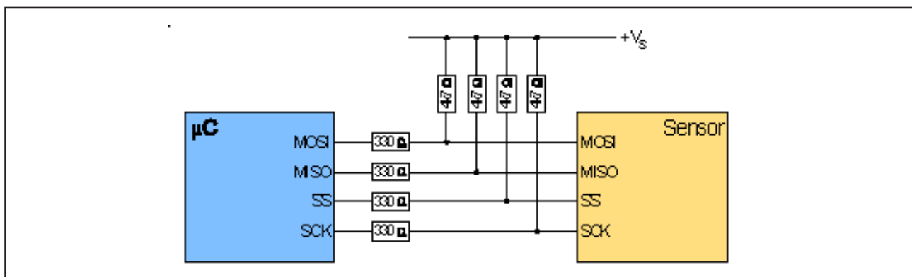
Bild 7: SPI-Bus Anwenderschaltung für HTD, HME- und HCE-Drucksensoren
