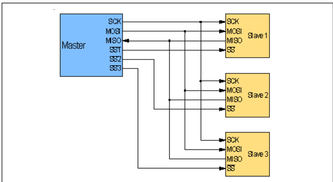
Bild 1: Beispiel eines SPI-Bus-Aufbaus mit einem Master und mehreren Slaves
